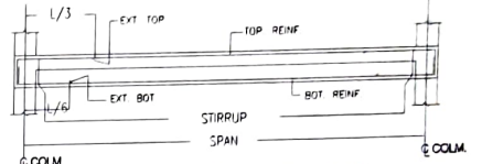
R.C. DET. OF BEAM CURTAILMENT SCALE - N.T.S.
