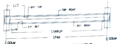
R.C. DET. OF BEAM CURTAILMENT SCALE - N.T.S.
