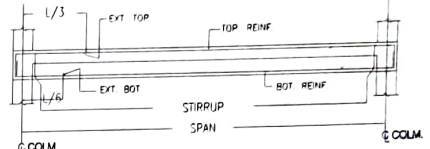
R.C. DET. OF BEAM CURTAILMENT SCALE - N.T.S.
