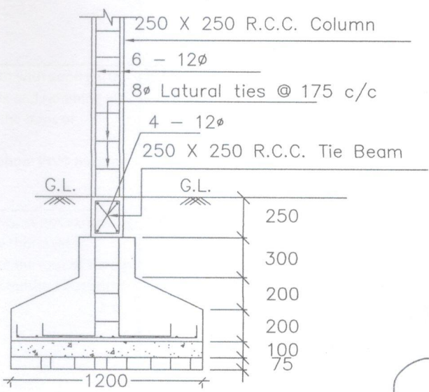
(SCALE - 1 : 25)
